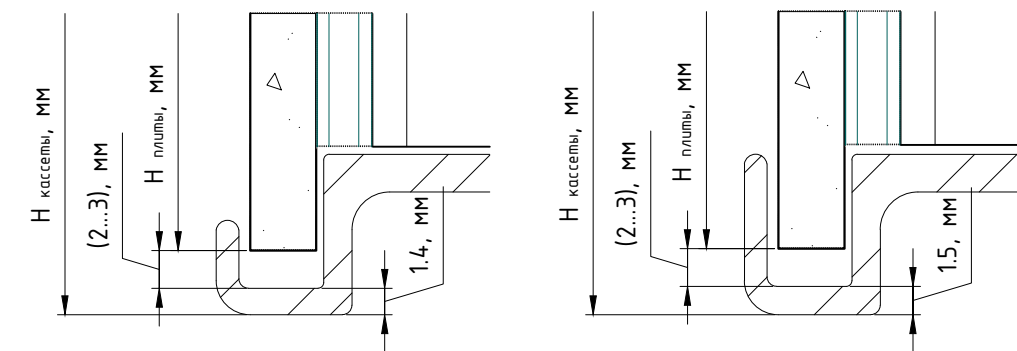
Узел №1 (увеличено)
