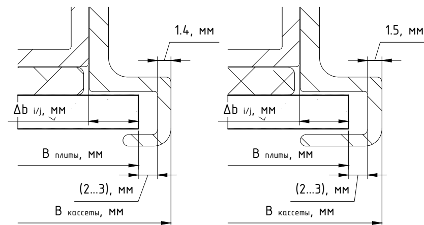
Узел №2 (увеличено)
