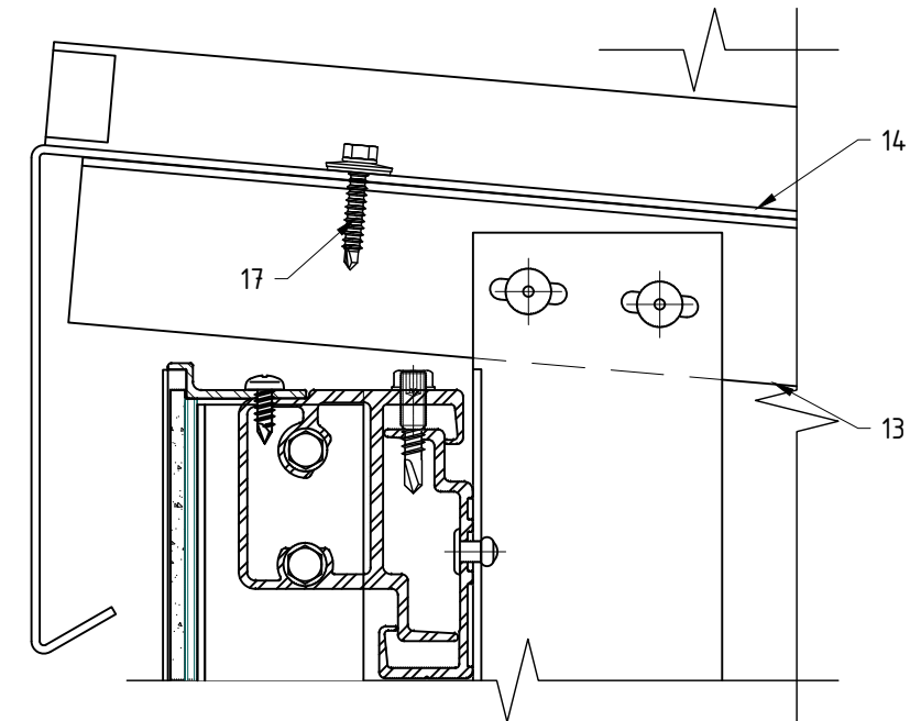
Вариант крепления парапетной крышки №3
