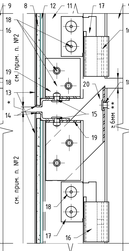
Фрагмент №1 (вариант с вертикальными несущими и горизонтальными поддерживающими профилями, для вертикального профиля в середине кассеты)
