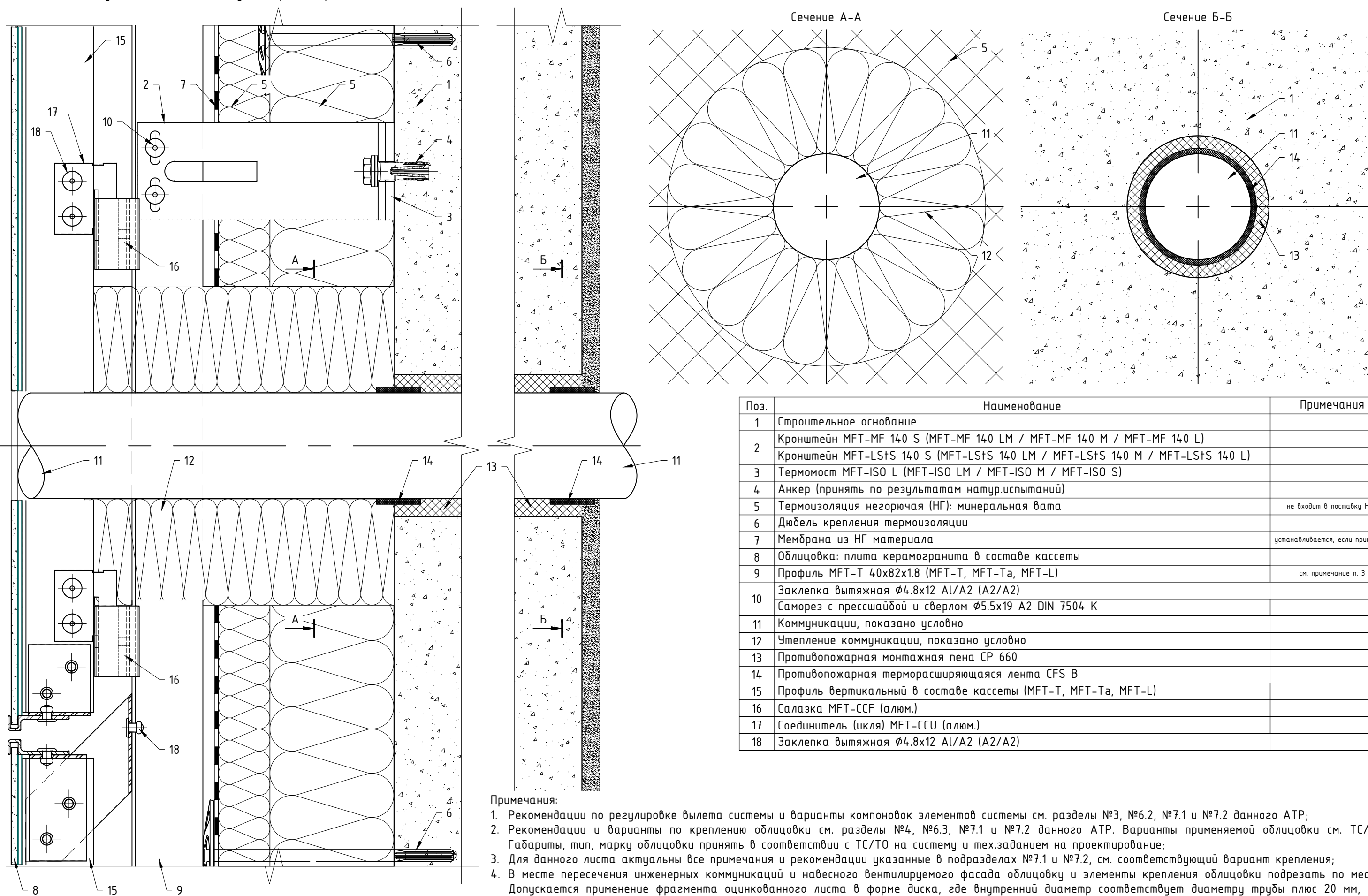
7.11. Ввод коммуникаций: элементы "Light", скрытое крепление на салазки.
